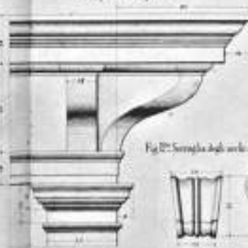
Fig. 18. Sezione della facciata, o sezione della parete.
